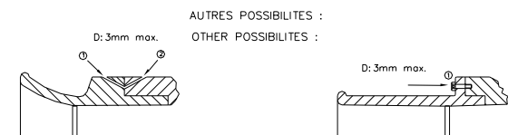
Dessin / Drawing 254-4
